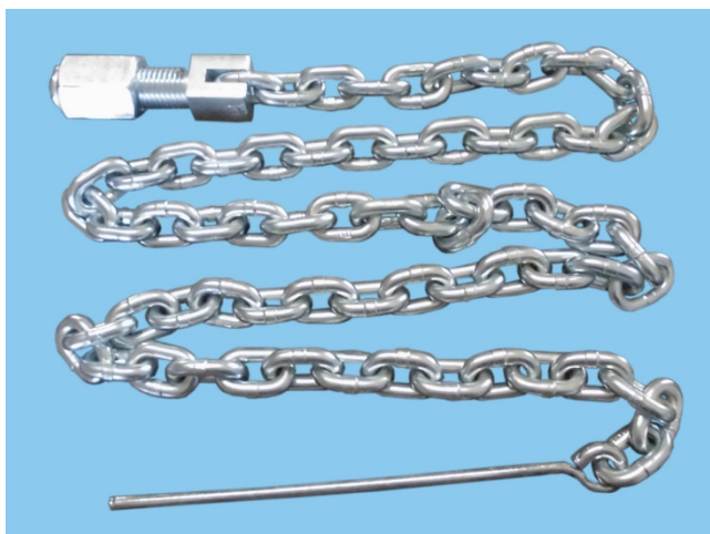
⑧締付ナット(④と一体型) (ガイド付き鎖+締め付けナット)
